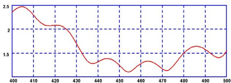
VSWR
